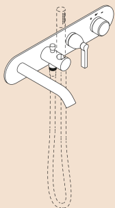
Gruppo termostatico ad incasso per vasca con deviatore e supporto per doccia / Recessed thermostatic bathtub taps set with diverter and hand-held shower support
