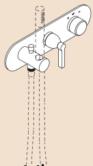
Gruppo termostatico a parete con deviatore e supporto doccia / Built-in thermostatic control with diverter and hand-held shower support
