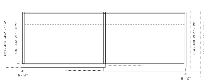
Sezione per anta WARM sp. 30 - th. 1 1/4"
