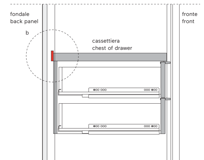
sezione struttura Tian Tian structure section
