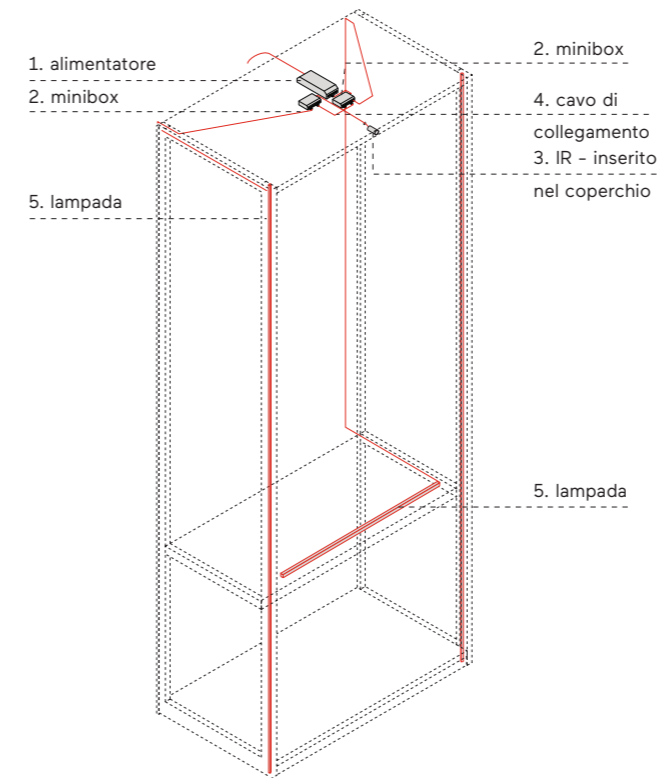
c. Illuminazione verticale e orizzontale con fianco telaio Horizontal and vertical lighting for frame side panel
