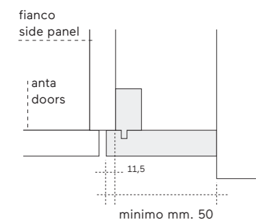
Fascia senza guarnizione Without rubber profile
