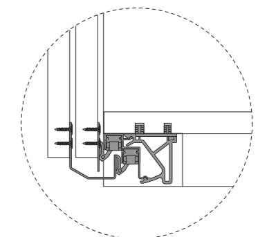
b. Sezione binario inferiore Section of lower rail
