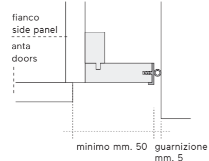
Sezione orizzontale soluzione battente, scorrevole, complanare
