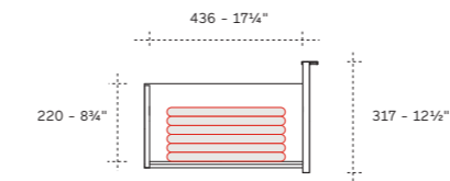
Cassetto frontale legno H 317 Wood drawer front H 12½"
