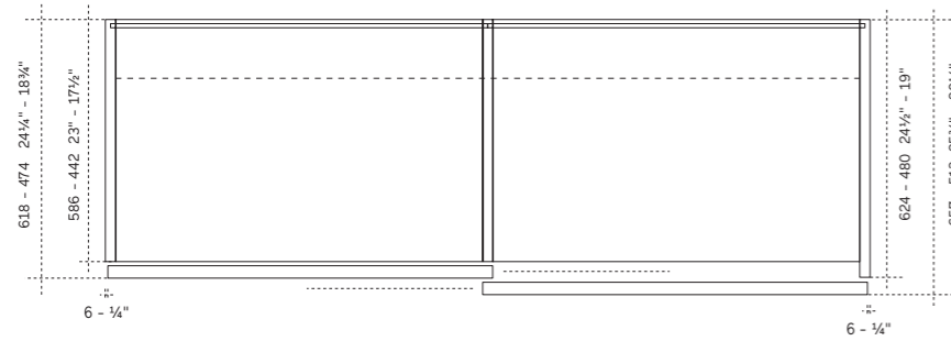
Sezione per anta PRIMA - TEXT - EMERY - ELLEVI sp. 25 - th. 1"
