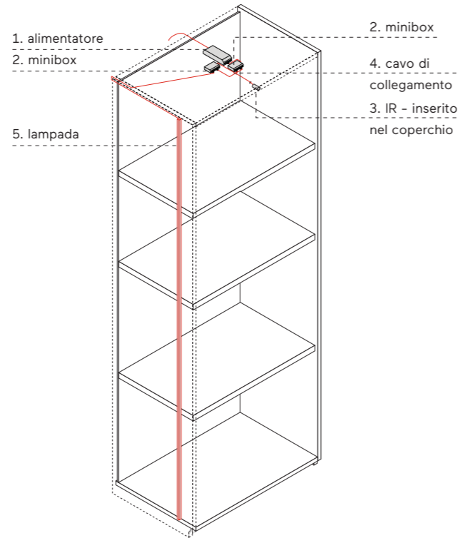
b. Illuminazione verticale con fianco in melaminico Vertical lighting for wood side panel
