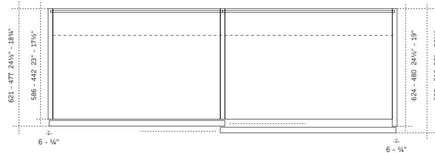
Sezione per anta NAICA sp. 28 - th. 1"
