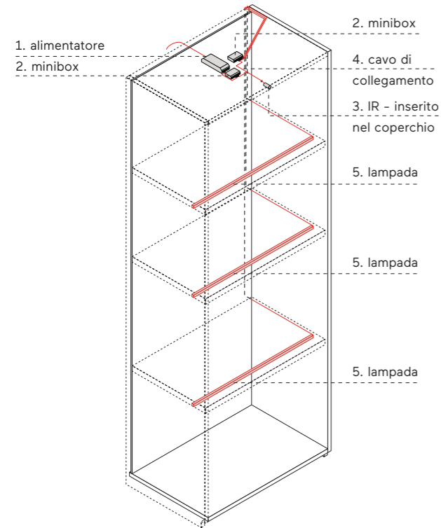
a. Illuminazione orizzontale con fianco in melaminico Horizontal lighting for wood side panel
