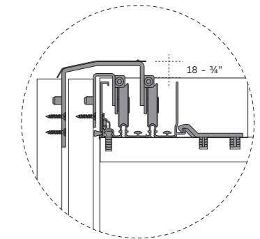
a. Sezione binario superiore Section of upper rail
