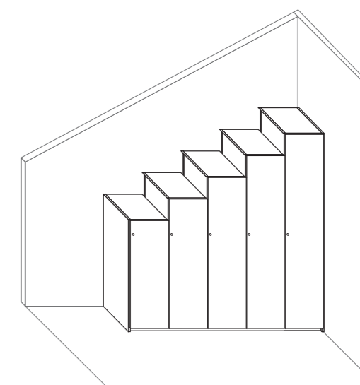
06 Soluzione a scaletta per mansarda Stair solution for attic Anta battente Hinged door
