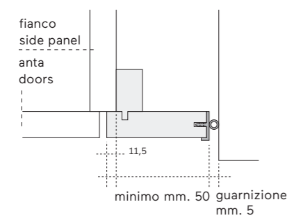
Sezione orizzontale soluzione battente
