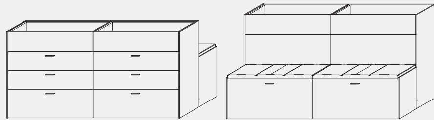
Fronte - Front L. 2180 H. 840 P. 952 W. 85¼" H. 33 D. 37½"
