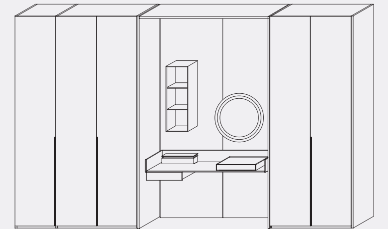
L. 4673 H. 2624 P. 586 W. 184" H. 103¼" D. 23"
