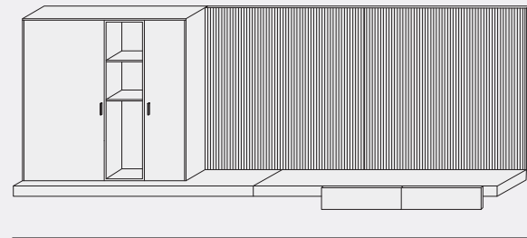
L. 3280 H. 1150 P. 510 W. 129¼" H. 45¼" D. 20"
