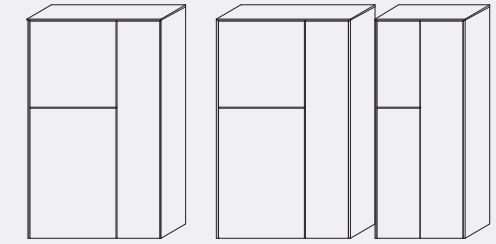
L. 832 – 832 – 562 H. 1360 P. 351 W. 32¼" – 32¼" – 22¼" H. 53½" D. 13¼"
