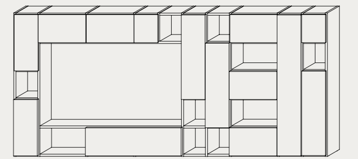
Pag. 60 –61 L. 2268 H. 2498 P. 366 W. 89¾" H. 98¾" D. 14½"
