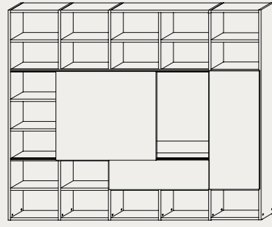
Pag. 68 –69 L. 2416 H. 2142 P. 346 W. 95" H. 84¼" D. 13½"
