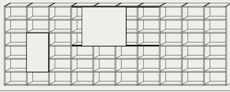
Pag. 26 –27 L. 5998 H. 2142 P. 346 W. 236¾" H. 84¾" D. 13½"
