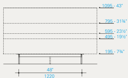
Composizione – Composition L. 1800 - 70 3/4"
