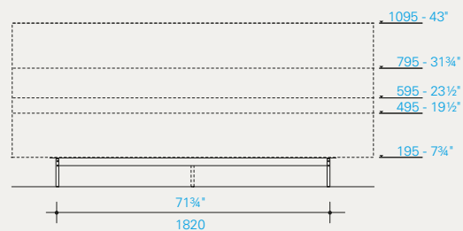
Composizione – Composition L. 2400 - 94 1/2"
