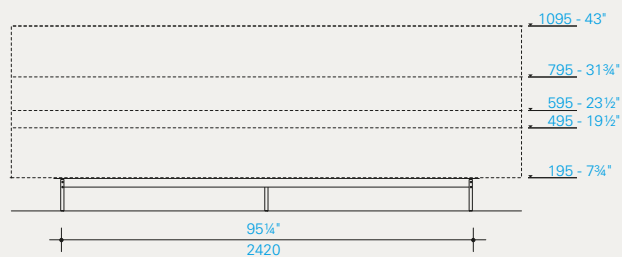
Composizione – Composition L. 3000 - 118"
