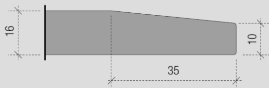
Sezione struttura / Structure section
