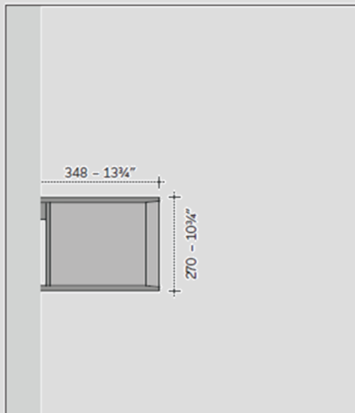
Sezione struttura / Structure section
