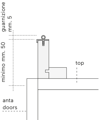
Sezione orizzontale soluzione battente
