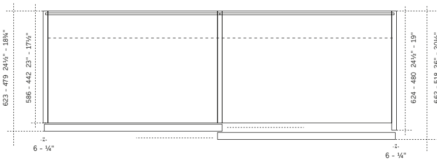
Sezione per ante WARM sp. 30 - th. 1 1/4"
