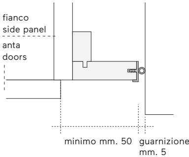
Sezione orizzontale soluzione battente, scorrevole, coplanare
