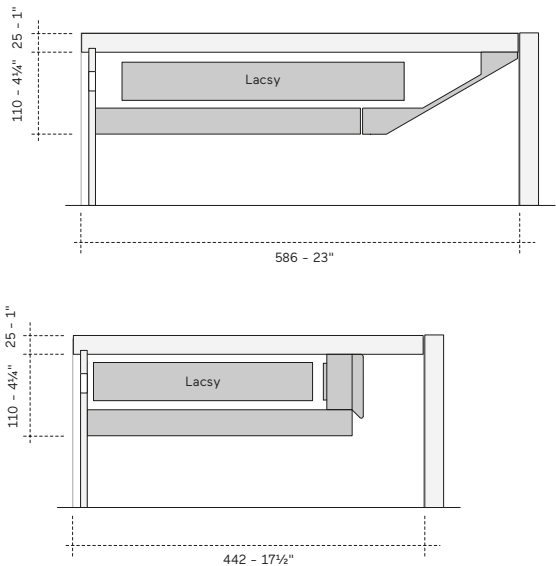
Sezione fianco Side section
