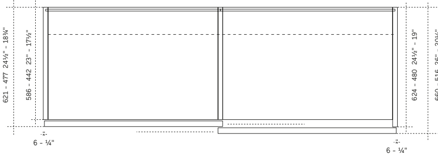
Sezione per ante NAICA sp. 28 - th. 1"
