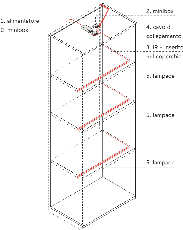
a. Illuminazione orizzontale con fianco in melaminico
