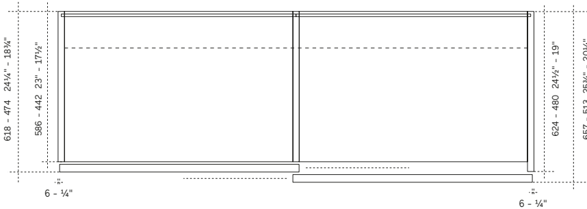
Sezione per ante PRIMA - TEXT - EMERY - ELLEVI sp. 25 - th. 1"
