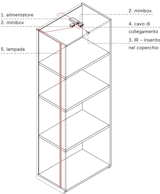
b. Illuminazione verticale con fianco in melaminico
