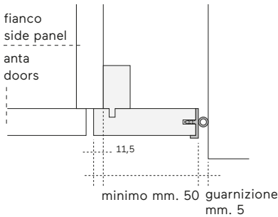
Sezione orizzontale soluzione battente
