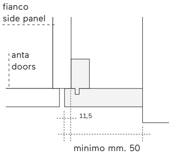
Fascia senza guarnizione Without rubber profile
